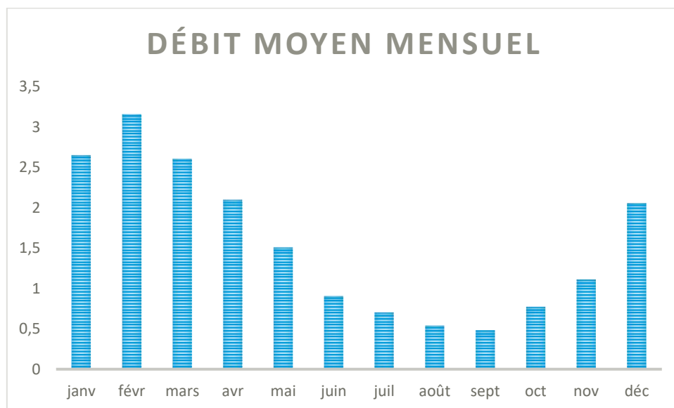
Figure n°16 : Graphique du débit moyen mensuel de la Douze à Cazaubon (Hydreau France)
