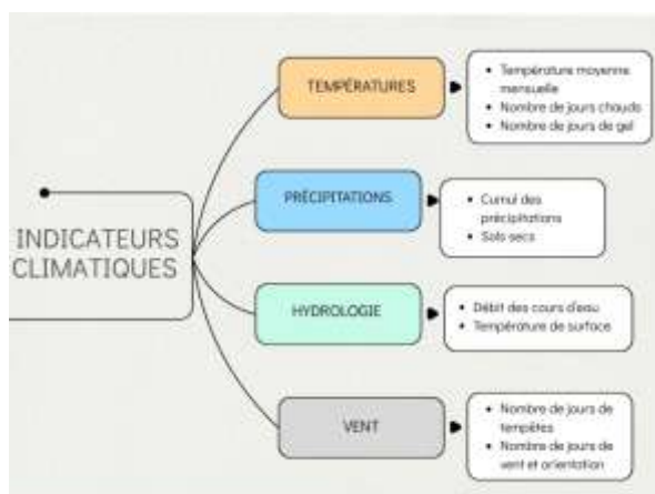
Figure n°3 : Schéma des indicateurs climatiques
